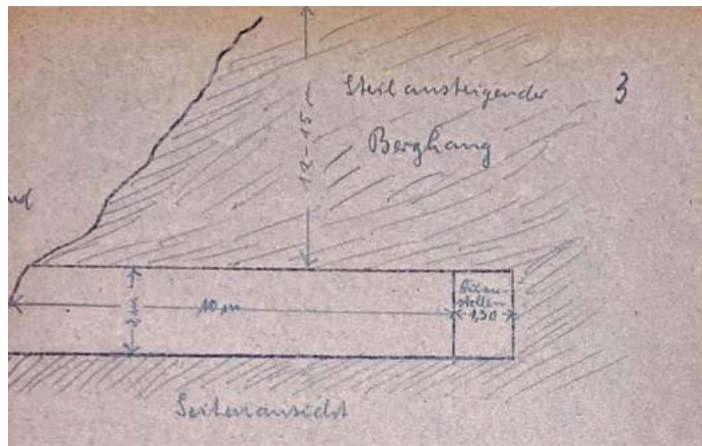
I Querschnitt der geplanten Stollenanlage am Mühlenberg/Elbkurhaus.
